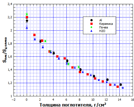
Рисунок 6. Графики экспериментальных зависимостей отношения темпов счета площади пика полного поглощения для энергии гамма-квантов 662 кэВ к площади комптоновской долины от толщины поглотителя для различных материалов (керамика, алюминий, почва, вода)
