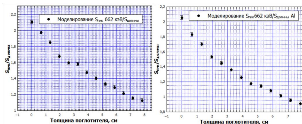
Рисунок 3. График зависимости отношение площади пика полного поглощения к площади долины от толщины поглотителя (керамика (а) и алюминий (б))
