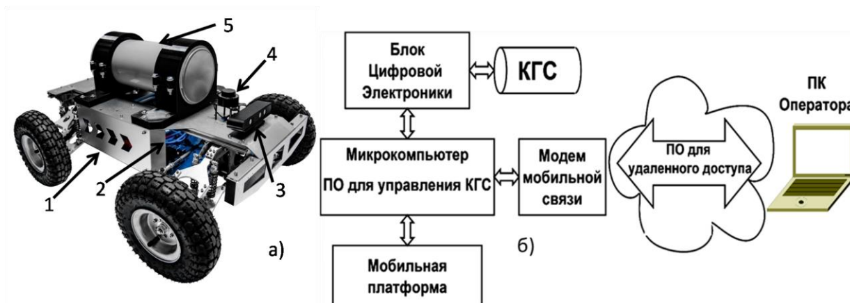
Рисунок 8. Беспилотный гамма-спектрометрический комплекс (а): 1 – мобильная платформа, 2 – блоки электроники, 3 – видеочкамера, 4 – LIDAR (лазерный дальномер), 5 – КГС; (б): блок-схема организации удаленной связи и управления БГСК
