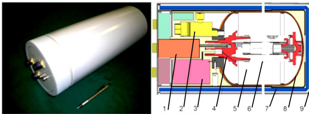
Рисунок 1. Фотография и схема КГС: 1 - зарядочувствительный усилитель, 2 - кран для наполнения рабочим веществом, 3 - источник питания, 4 - керамический гермоввод, 5 - ионизационная камера, 6 - экранирующая сетка, 7 - тефлоновая изоляция, 8 - стальной корпус с композитным покрытием, 9 - внешний защитный корпус.
