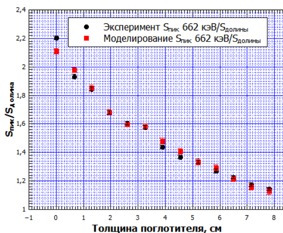
Рисунок 7. График зависимости отношения темпа счета площади пика полного поглощения для энергии гамма-квантов 662 кэВ к темпу счета площади комптоновской долины от толщины поглотителя (керамика)
