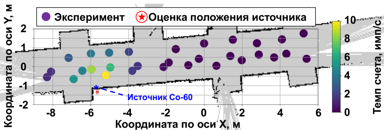
Рисунок 12. Распределение темпов счета и положение источника на карте для анализа пиков 1173 кэВ и 1332 кэВ
