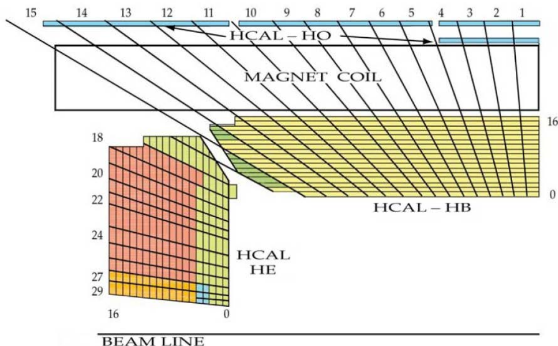
Рис. 1.11. Схема сегментации башен в центральном (HB), торцевом (HE) и внешнем (HO) адронных калориметрах (показана область отрицательных \eta ).
