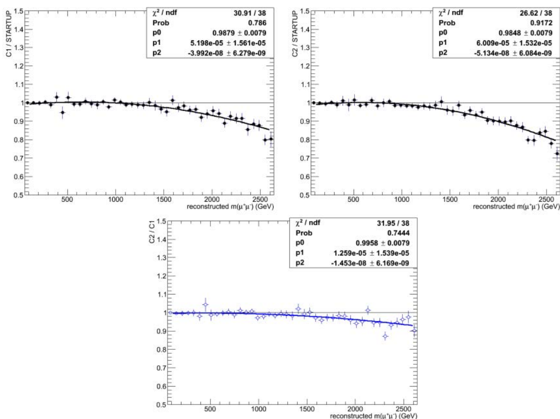
Рис. 6.157. Отношение числа фоновых событий в зависимости от массы пары для различных сценариев пространственной невыравненности детекторных систем: C1/STARTUP , C2/STARTUP и C2/1 [81].
