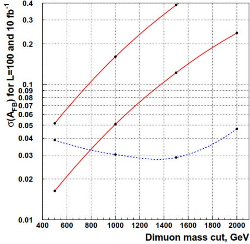
Рис. 3.76. Статистические ошибки измерения асимметрии A_{FB} в разных областях инвариантной массы пары мюонов m_{\mu\mu} для интегральной светимости: (нижняя красная кривая) 100 фбн -1 (верхняя красная кривая) 10 фбн -1 . Систематические ошибки (синяя кривая) преимущественно определяются вариациями ошибки определения направления движения кварка вследствие неопределенностей PDF семейства STEQ61 [62].
