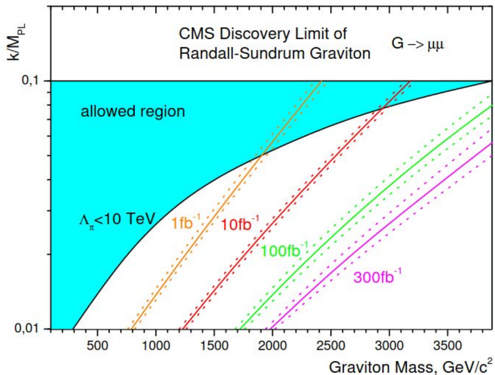
Рис. 4.104. Ожидаемые экспериментальные ограничения в пространстве параметров (\kappa/M_{5D}, m_{G_{KK}}) с учетом всех систематических погрешностей [4, 67, 50]. НДС учтен в сценарии First Data. Также приведены теоретические ограничения.
