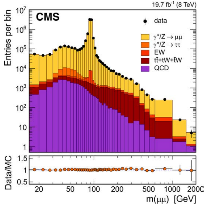
Рис. 5.125. Распределения событий по инвариантной массе пар мюонов при \sqrt{s} = 8 ТэВ (точки) [72]. Показаны результаты моделирования сигнала ( \mu^+\mu^- ) и вклад доминирующих фоновых процессов (гистограммы). Сигнал смоделирован с учетом NNLO-вкладов (POWHEG и FEWZ). Электрослабые процессы включают парное рождение калибровочных бозонов и события W + jet . Фон КХД оценен методом КНД.
