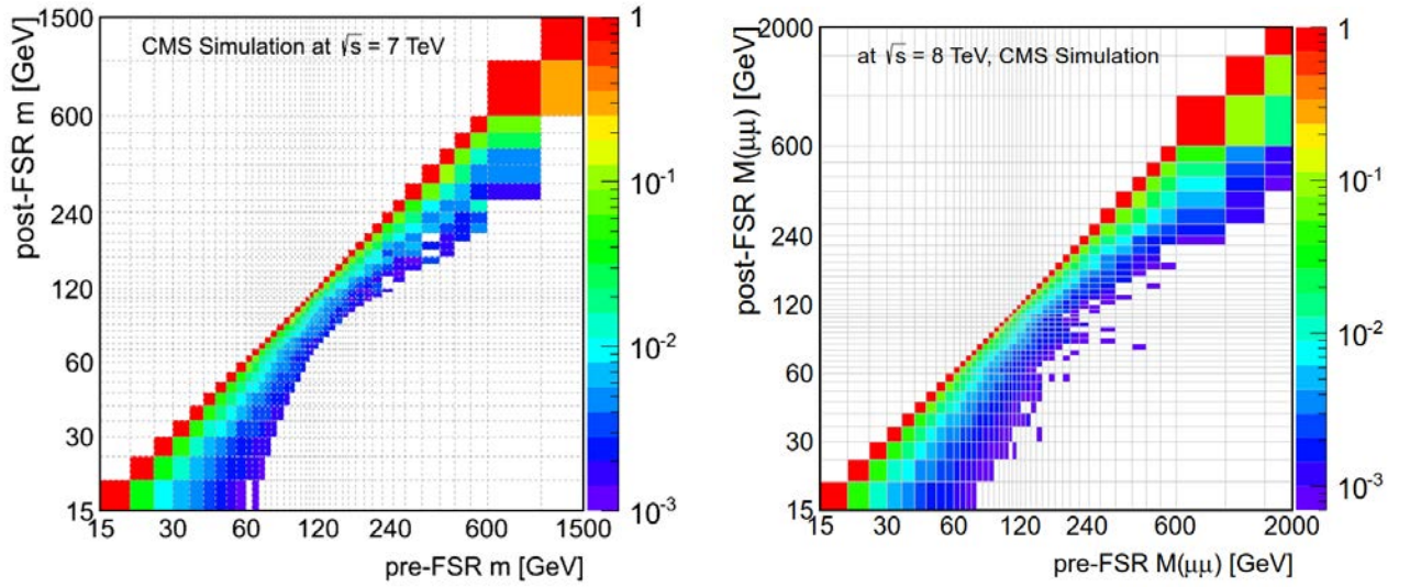
Рис. 5.134. Матрица отклика для учета FSR при \sqrt{s} = (слева) 7 ТэВ и (справа) 8 ТэВ.
