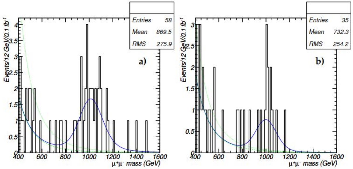
Рис. 4.108. Распределения событий по m_{\mu\mu} (гистограммы) в соответствии с \mathcal{L}_{\text{int}} = 100 пбн ^{-1} для нового калибровочного бозона (слева) Z'_{SSM} и (справа) Z'_{\psi} с массой 1000 ГэВ/ c^2 [53, 54]. Сплошными линиями приведены результаты аппроксимации ММП функциями правдоподобия для сигнала и фона (синяя линия) и только для фона (зеленая линия).
