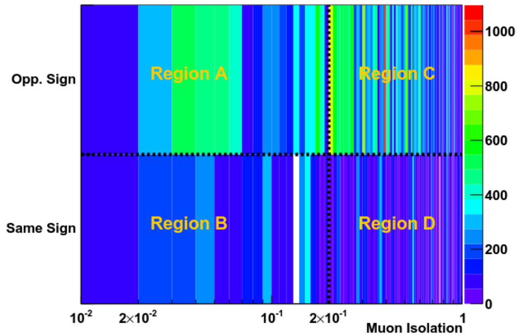
Рис. 5.122. Двумерный плот зависмости числа событий от заряда мюонов и величины относительного критерия изолированности I_{rel}^{comb} для процессов КХД: область A — сигнальная с мюонами преимущественно из процессов Дрелла-Яна, B — с преимущественно фоновыми событиями, C и D — практически все события фоновые.
