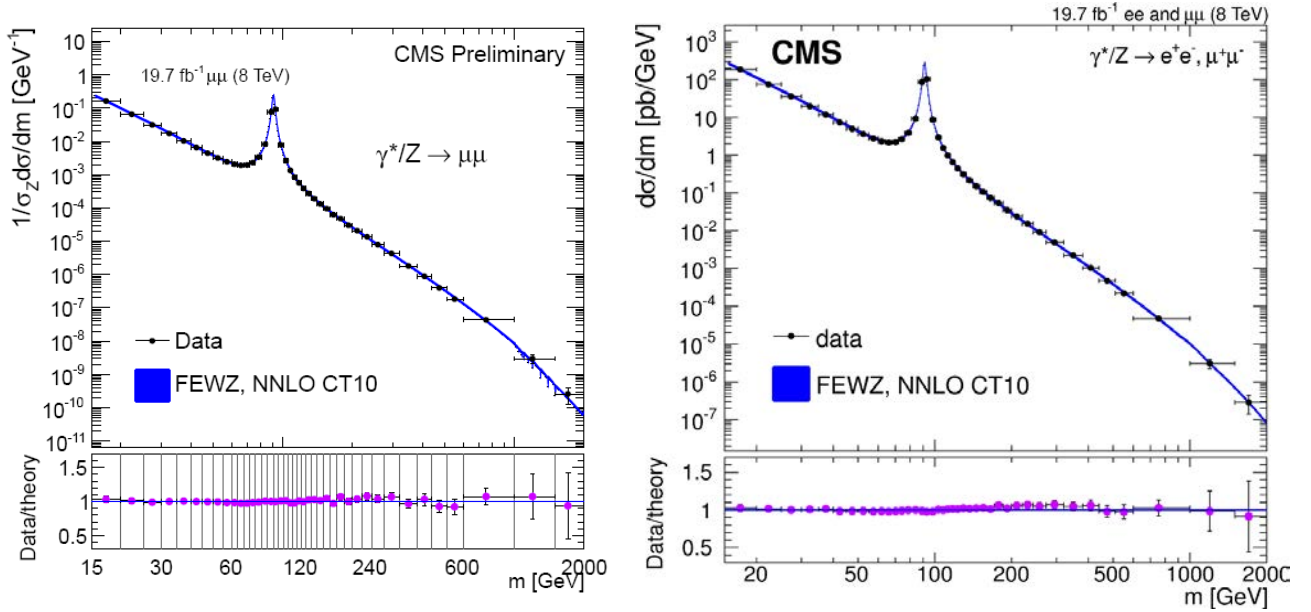
Рис. 5.136. Дифференциальное сечение 1/\sigma_Z d\sigma/dm рождения пар (слева) мюонов и (справа) лептонов ( e^+e^- и \mu^+\mu^- ) в процессе Дрелла–Яна при \sqrt{s} = 8 ТэВ [72]. Приведено отношение экспериментальных данных и предсказаний СМ в NNLO КХД и NLO ЭС. Вычисления сделаны в FEWZ3.1 с PDF CT10. Приведены квадратично просуммированные статистические и систематические ошибки. Область теоретических погрешностей включает также квадратично просуммированные статистическую погрешность вычисления в FEWZ3.1 и ошибку вычисления, связанную с PDF. Значение критерия согласия результатов измерения и теоретических предсказаний \chi^2_{n.d.f.} = 1.0 (с n.d.f. = 40).
