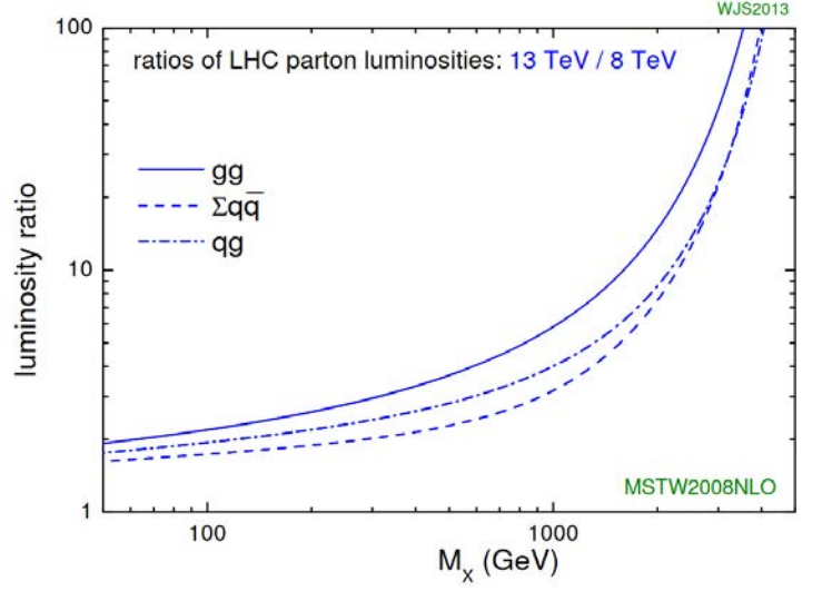
Рис. 5.118. Соотношение партонных светимостей при \sqrt{s} = 13 и 8 ТэВ.
