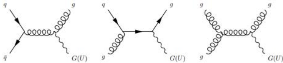
Рис. 4.79. Процессы реального рождения ADD-гравитона q\bar{q} \rightarrow gG_{\text{KK}} , qg \rightarrow gG_{\text{KK}} , gg \rightarrow gG_{\text{KK}} .
