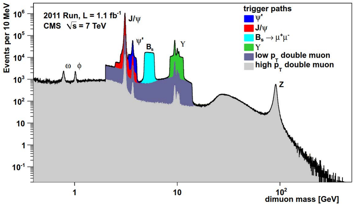
Рис. 5.117. Резонансы СМ в спектре инвариантных масс пар мюонов при \sqrt{s} = 7 ТэВ. Статистика соответствует \mathcal{L}_{\text{int}} = 1.1 \text{ фбн}^{-1} (примерно два месяца набора данных в 2011 г.).
