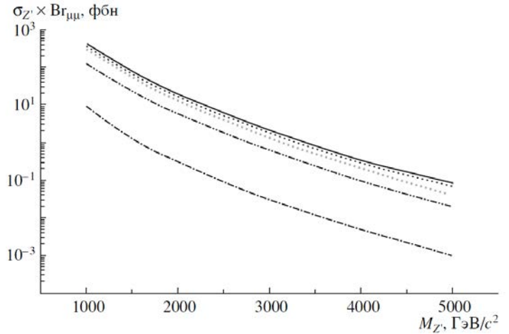
Рис. 4.105. Зависимость сечения рождения мюонов из распадов Z' согласно SSM, LRM, \chi^- и \psi -моделям, а также для процесса Дрелла-Яна (кривые сверху вниз соответственно) в pp -соударениях при \sqrt{s} = 14 ТэВ [69].
