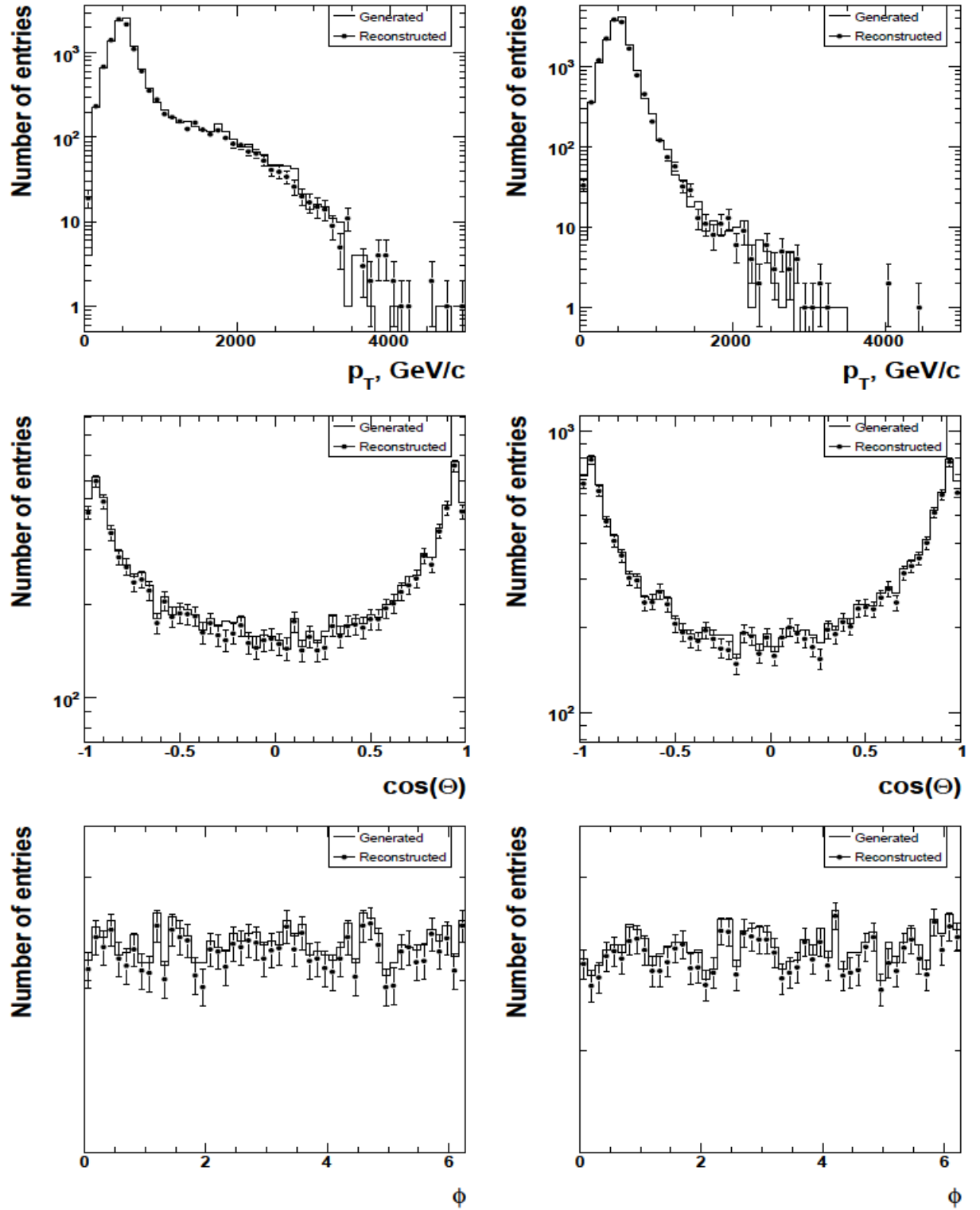
Рис. 4.85. Распределения смоделированных (гистограммы) и реконструированных (точки) событий рождения пар мюонов по p_T , \cos \theta , \phi в сценарии ADD с фундаментальным масштабом M_S = 7 ТэВ и числом дополнительных измерений (слева) n = 3 и (справа) n = 6 [63]. Учтена остаточная невыравненность детекторных систем в соответствии с долгосрочным сценарием Long Term.
