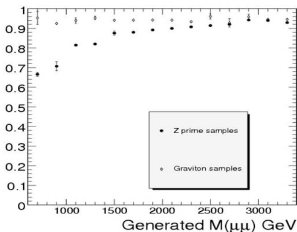
Рис. 4.91. Эффективность аксептанса для событий распада RS1–гравитона и нового калибровочного бозона Z' на пару мюонов [67].
