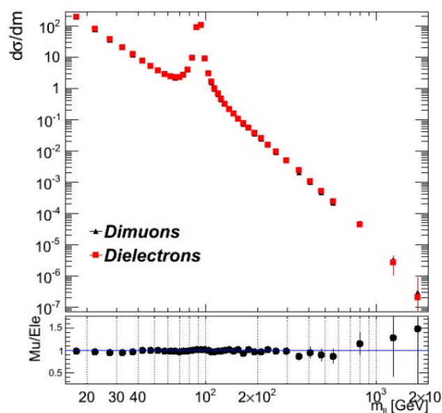
Рис. Г.2. Сравнение дифференциальных сечений d\sigma/m рождения пар мюонов ( \mu^+\mu^- ) и электронов ( e^+e^- ) в процессе Дрелла-Яна при \sqrt{s} = 8 ТэВ. В нижней части рисунка представлено отношение измеренного сечения в двух независимых каналах. Погрешности экспериментальных данных представляют собой квадратично просуммированные статистические и систематические ошибки.
