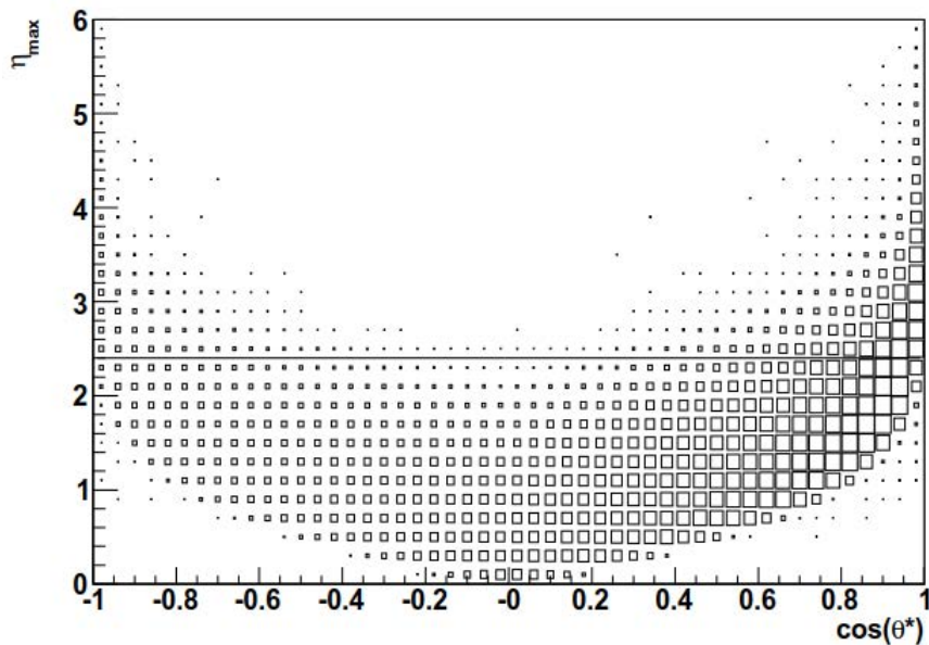
Рис. 3.73. Двумерное распределение числа событий МК с m_{\mu\mu} \geq 1 ТэВ/ c^2 по \cos \theta^* и максимальному значению псевдобыстроты мюонов в событии \eta_{max} . Линия \eta_{max} = 2.4 соответствует аксептансу установки CMS [62].
