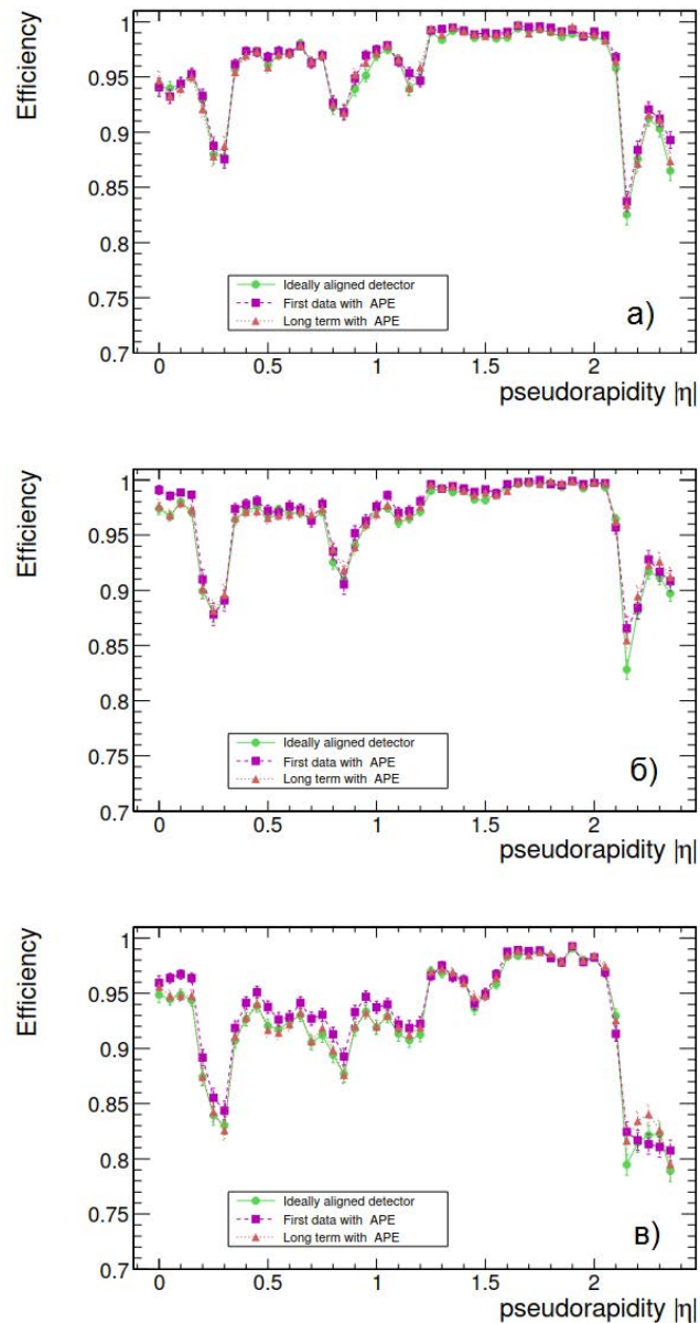
Рис. 2.43. Эффективность триггера Level-3 для идеального выравнивания и различных сценариев невыравнивания. Приведены результаты для одиночных мюонов с поперечными импульсами (а) 10 ГэВ/с, (б) 100 ГэВ/с и (в) 1000 ГэВ/с [52].
