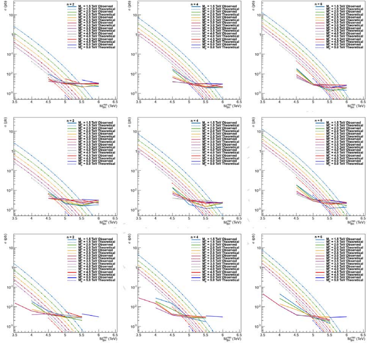
Рис. Д.2. Верхние пределы (95% CL) на сечение рождения квазиклассических МЧД в зависимости от минимальной массы M_{\text{BH}}^{\min} для числа дополнительных измерений n = 2, 4, 6 и различных сценариев: (верхний ряд) шварцшильдовская МЧД, (средний ряд) керровская МЧД и (нижний ряд) керровская МЧД с 10% потерями массы и момента импульса без конечного остатка. Сечения приведены для значений фундаментального масштаба M_D от 1.5 до 5.0 ТэВ. Также показаны теоретические сечения (пунктирные линии), рассчитанные с помощью генератора CHARYBDIS2 . Из работы [89].
