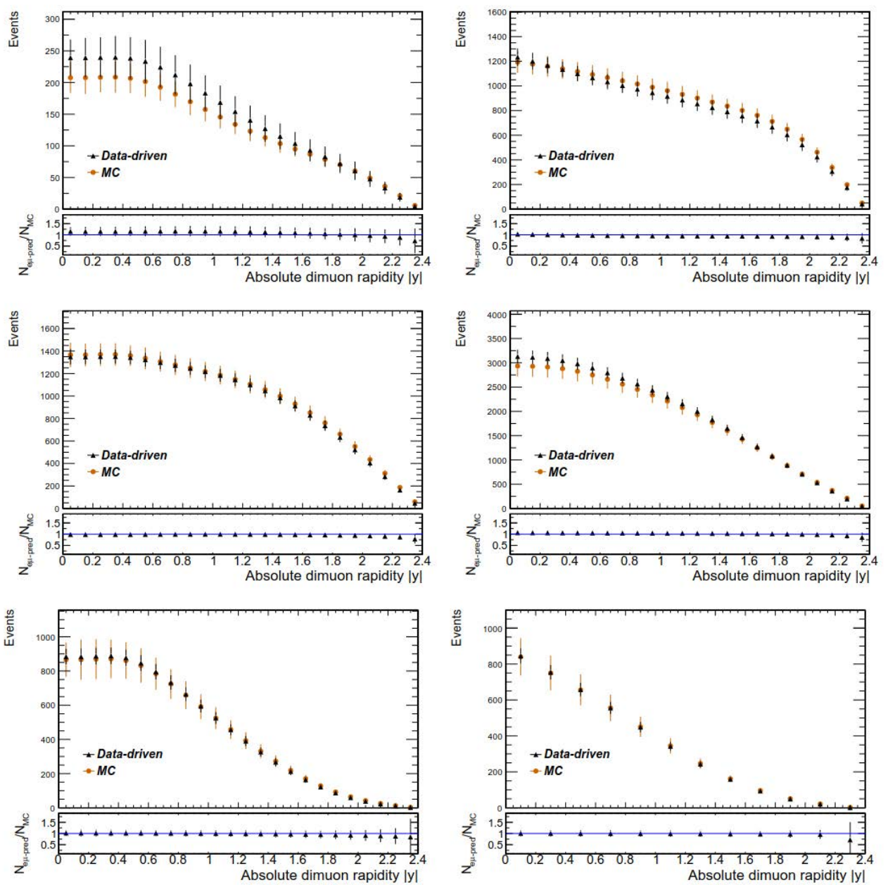
Рис. 5.124. Зависимость числа фоновых событий при \sqrt{s} = 7 ТэВ, оцененных e\mu -методом, в сравнении с предсказаниями МК для различных интервалов m_{\mu\mu} : (а) 20 < m_{\mu\mu} < 30 ГэВ/ c^2 , (б) 20 < m_{\mu\mu} < 45 ГэВ/ c^2 , (в) 45 < m_{\mu\mu} < 60 ГэВ/ c^2 , (г) 60 < m_{\mu\mu} < 120 ГэВ/ c^2 , (д) 120 < m_{\mu\mu} < 200 ГэВ/ c^2 , (е) 200 < m_{\mu\mu} < 1500 ГэВ/ c^2 . Учтены статистические и систематические ошибки.
