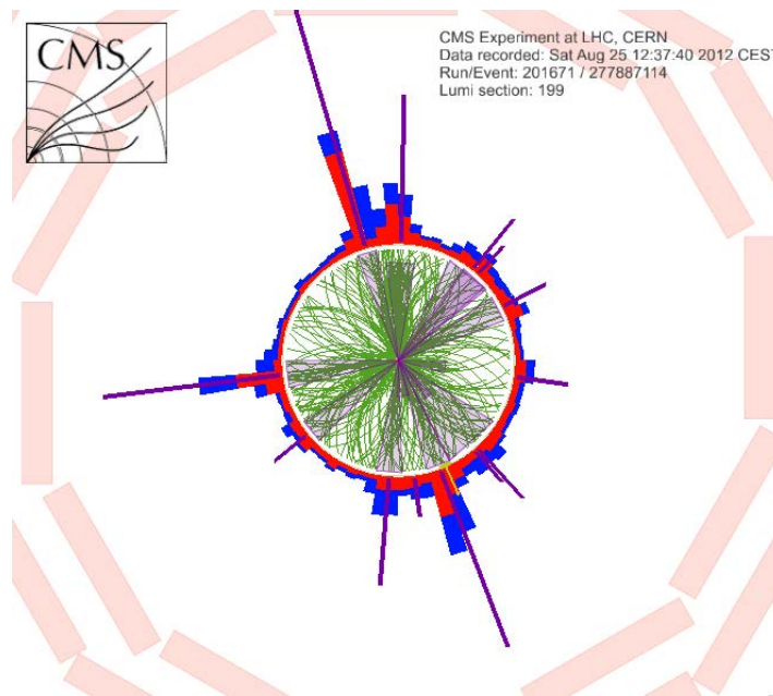
Рис. 7.165. Визуализация реального события – кандидата в МЧД с 13 объектами в конечном состоянии, S_T = 2.1 ТэВ, \sqrt{s} = 8 ТэВ в с.ц.м. (2012г).
