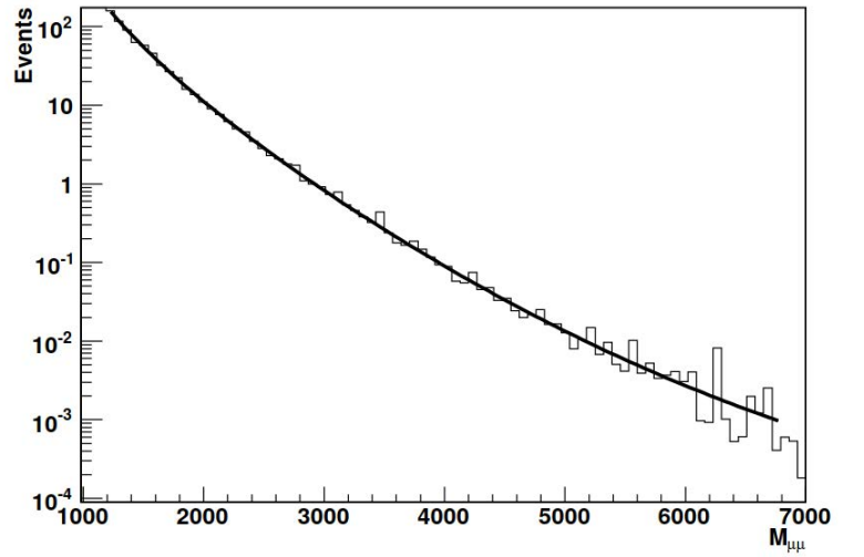
Рис. 4.97. Распределение реконструированных событий МК процесса Дрелла–Яна по m_{\mu\mu} . Аппроксимация сделана с помощью (4.61) [67].
