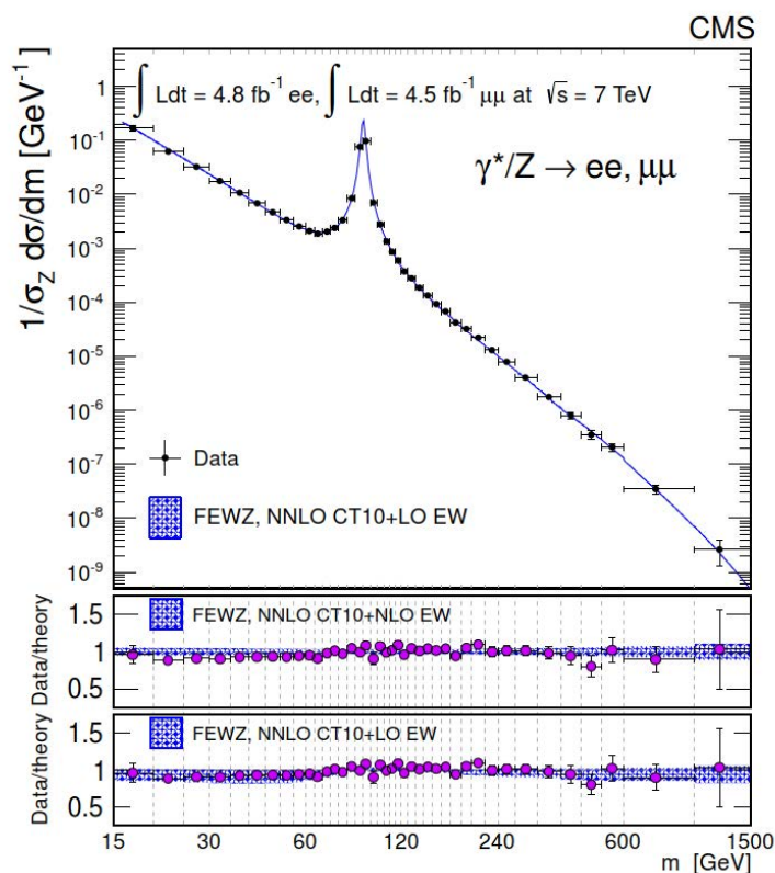
Рис. Г.3. Дифференциальное сечение 1/\sigma_Z d\sigma/dm рождения пар мюонов и лептонов ( e^+e^- и \mu^+\mu^- ) в процессе Дрелла-Яна при \sqrt{s} = 7 ТэВ [71]. Приведено отношение экспериментальных данных и предсказаний СМ в NNLO КХД и NLO ЭС. Вычисления сделаны в FEWZ3.1 с PDF CT10. Приведены квадратично просуммированные статистические и систематические ошибки. Область теоретических погрешностей включает также квадратично просуммированную статистическую погрешность вычисления в FEWZ3.1 и ошибку вычисления, связанную с PDF. Значение критерия согласия результатов измерения и теоретических предсказаний \chi^2_{n.d.f.} = 1.1 (с n.d.f. = 40).
