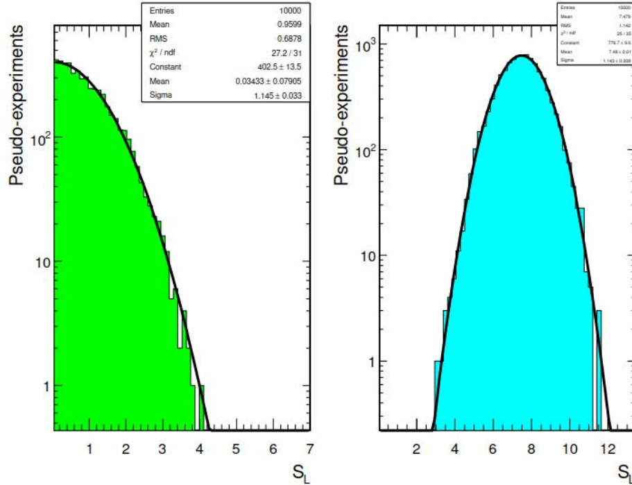
Рис. 4.99. Распределение значений оценщика S_L , полученное в 10^4 псевдоэкспериментах для интегральной светимости 100 фбн -1 , для случая (слева) отсутствия сигнала (только события Дрелл–Яна) и (справа) сигнальных событий рождения RS1–гравитона с массой 1500 ГэВ/ c^2 и c = 0.01 [67].
