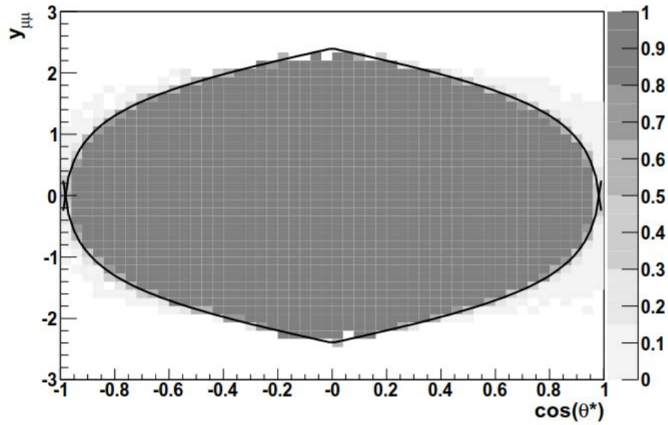
Рис. 3.72. Вероятность попадания обоих мюонов в аксептанс установки |\eta| \leq 2.4 в зависимости от \cos \theta^* и быстроты пары мюонов для области инвариантных масс m_{\mu\mu} \geq 1 ТэВ/ c^2 [62].
