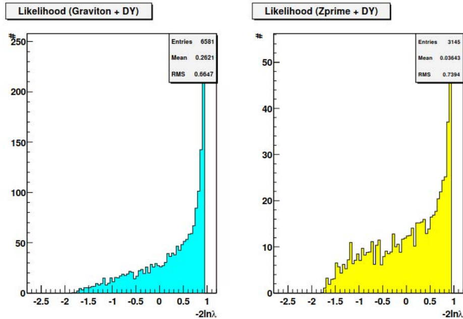
Рис. 4.112. Вклады в тестовую статистику (4.69) независимых событий рождения (слева) RS1-гравитона и (справа) нового калибровочного бозона Z' с массой 1000 ГэВ/ c^2 [67]. Учен вклад фоновых событий от процесса Дрелла–Яна.
