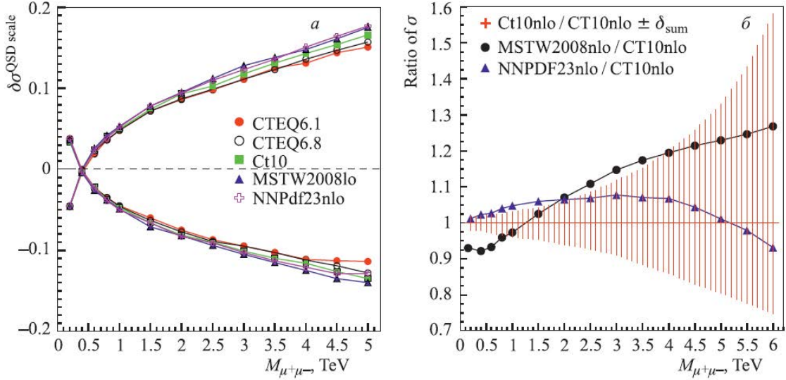
Рис. 3.67. (а) Зависимость относительных погрешностей вычисления сечения процесса Дрелла–Яна для LHC, связанных с неопределенностью шкалы факторизации, от инвариантной массы пары мюонов. (б) Сечения процесса Дрелла–Яна для CT10, MSTW2008, NNPDF23nlo, нормированные на аналогичные сечения для CT10. Приведен коридор комбинированных ошибок для CT10 [59].
