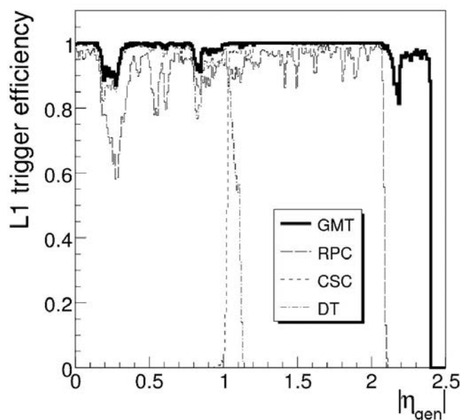
Рис. 2.38. Эффективность глобального мюонного триггера первого уровня (сплошная кривая) в зависимости от псевдобыстроты \eta перед применением критериев качества трека и наложении порогов обрезания на p_T . Также рассмотрены эффективности региональных триггеров подсистем DT, CSC и RPC (соответственно, штрихпунктирная, пунктирная и штриховая линии) [3].
