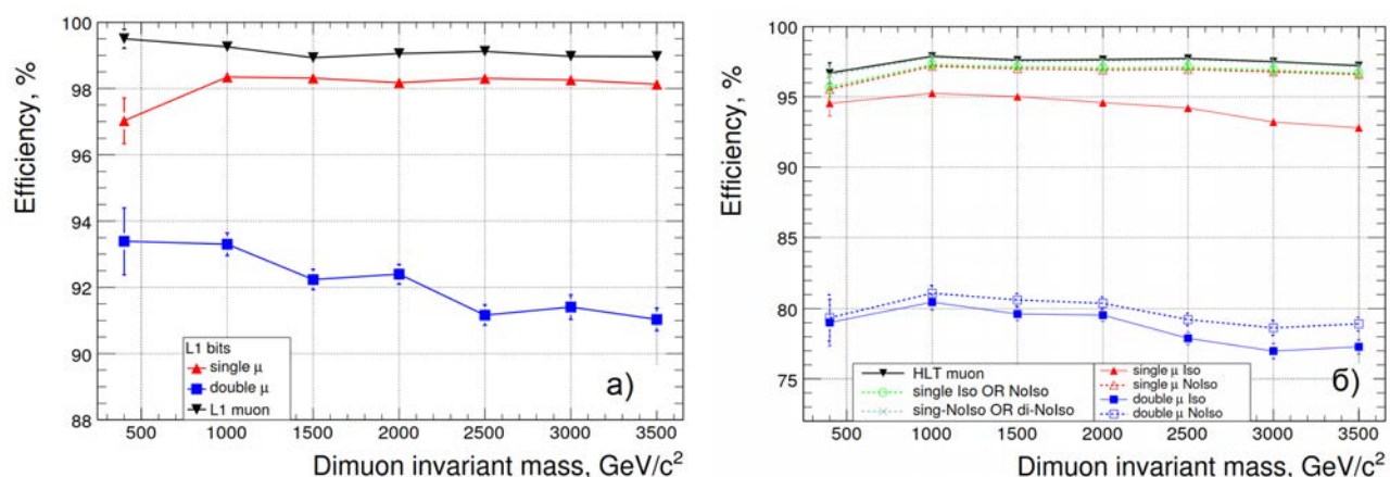
Рис. 2.40. Эффективность регистрации событий с парой мюонов триггером (а) Level-1 и (б) HLT. Рассмотрены случаи триггера на одиночный мюон, пару мюонов и их комбинации при \mathcal{L} = 10^{32} см -2 с -1 [54].
