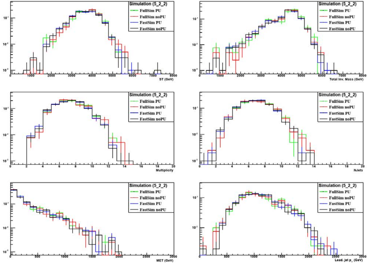
Рис. 7.167. Сравнение «отклика» детекторных систем CMS на сигнал образования МЧД для полного и быстрого моделирования на примере распределений числа событий по величине S_T , полной инвариантной массе, множественности, числу струй, потерянной энергии и поперечному импульсу лидирующей струи [89]. В качестве сигнала использовалось рождение МЧД с M_D = 1.5 ТэВ, M_{\text{ВН}}^{\text{min}} = 4.5 ТэВ/ c^2 и n = 2 (BLACKMAX). Рассмотрены случаи с учетом и без учета наложения событий (pile-up).
